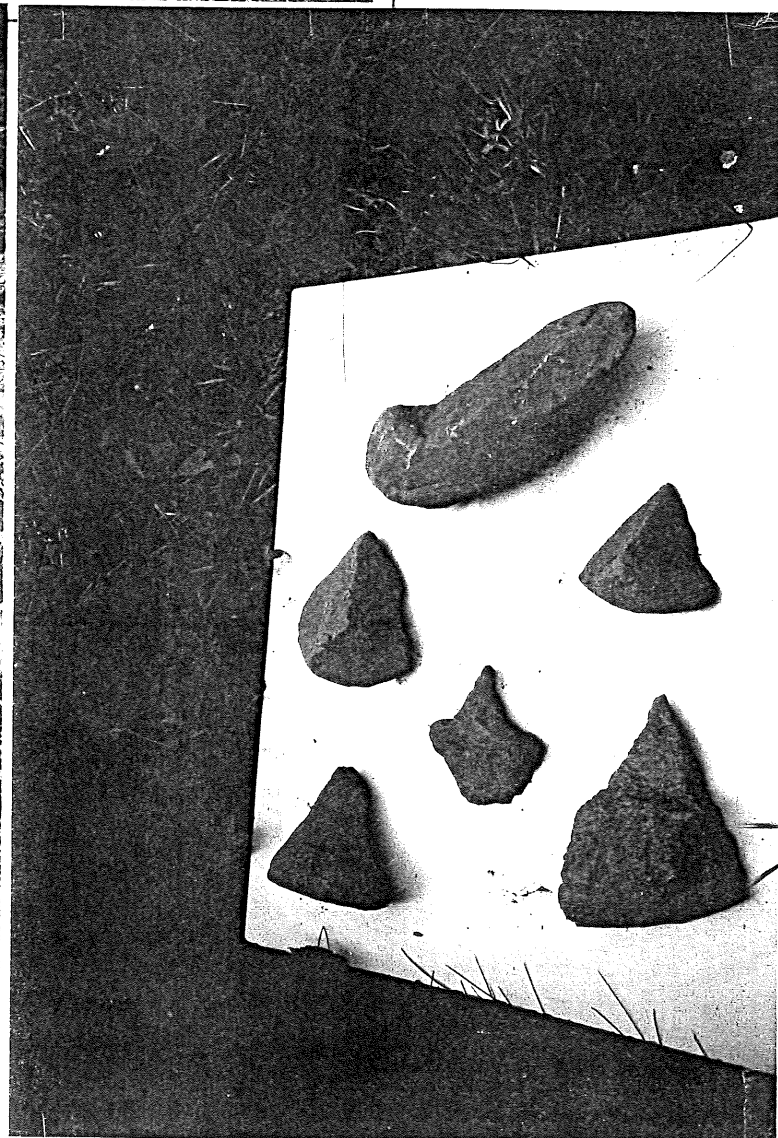
DURANTE UNO SCAVO PER LA POSA DI UN COLLETTORE DELLA PROFONDITÀ DI CIRCA 7 o 8 M., SI È EVIDENZIATA UNA STRATIFICAZIONE GEOLOGICA MOLTO INTERESSANTE. SUL FONDO SI È NOTATA UNA CERCHIATURA DI CIOTOLI LI ANDATA PERDUTA DURANTE I LAVORI, E DEI SASSI SCHEGGIATI A PUNTA DEL TIPO "CHOPPER" o "CHOPPING TOOL" DA ME RECUPERATI (FOTO SOPRA) E RESIDUI DI LAVORAZIONE DI SELCI
