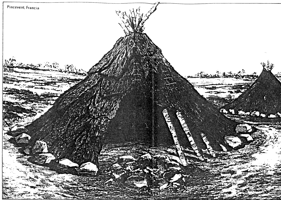
LA CERCHIATURA DI CIOTOLI RILEVATA A UNA PROFONDITÀ DI CIRCA 7 M. NEL SEDIMENTO DI GHIAIETTO SOTTO IL SEDIMENTO DI ARGILLA CHE SEMBRA DEL PERIODO INTERGLACIALE RISS WURM (L'IPOTESI È PERSONALE) SEM- BRA STATA UTILIZZATA PER ANCORAGGIO DI PELLI DI UNA TENDA PREISTORICA SIMILARE ALLA RICOSTRUZIONE DELLA TENDA PALEOLITICA DELLA REGIONE DI PIN- CEVENT FRANCIA (DISEGNO SOPRA).
