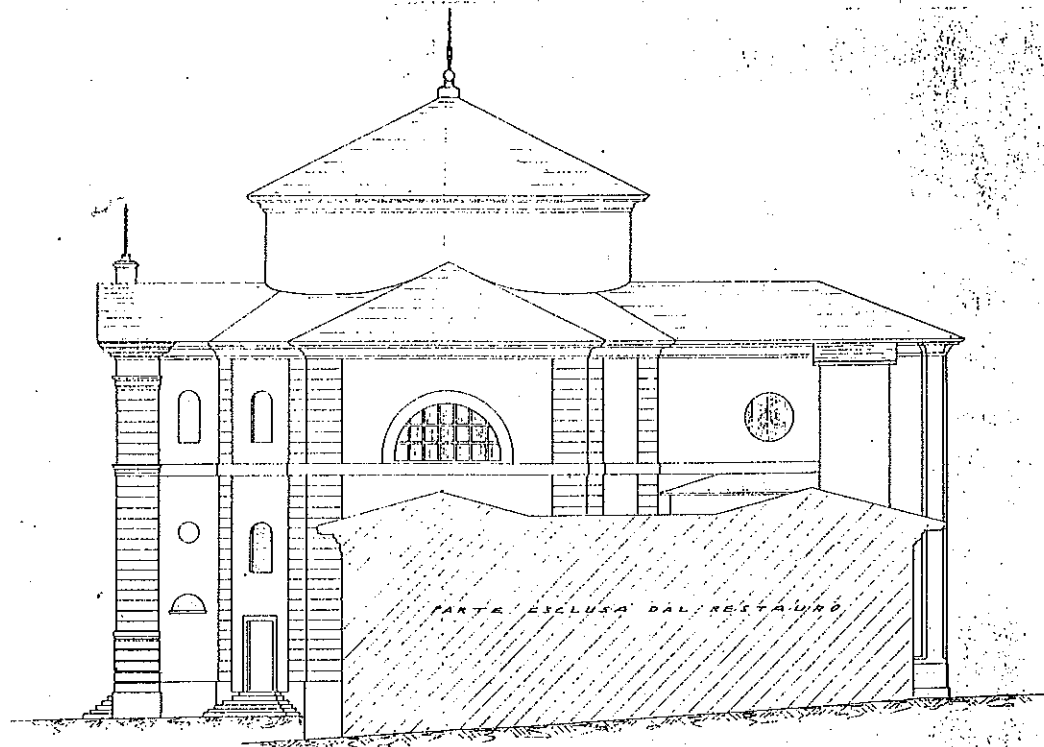
PROSPETTI DEL LATO SETTENTRIONALE E DI QUELLO MERIDIONALE
