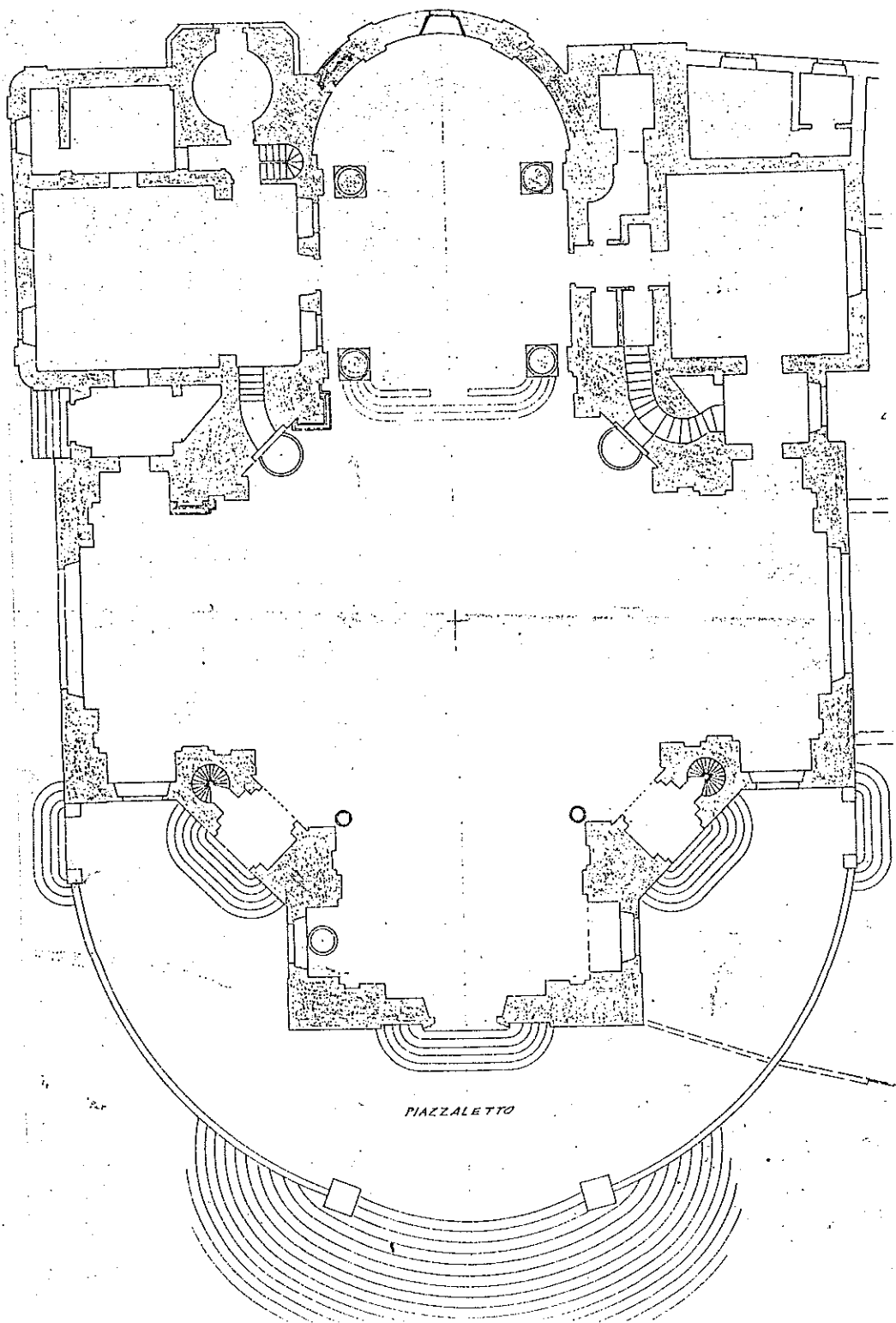
PLANIMETRIA DELLA PARROCCHIALE DI GORLA MAGGIORE NEL 1960
