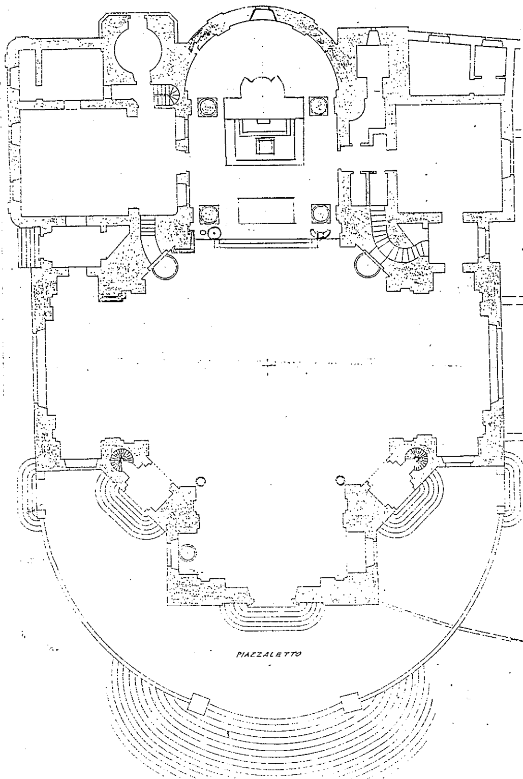
DISPOSIZIONE DEI POLI LITURGICI - PIANTA - DOPO IL CONCILIO VATICANO II
