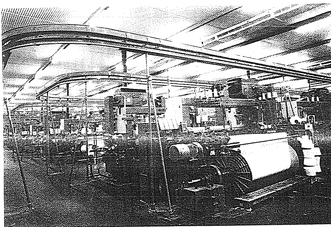
GE.TE.CA S.r.l. - Stabilimento di Castellanza - Nuova Sala Telai ad aria.
