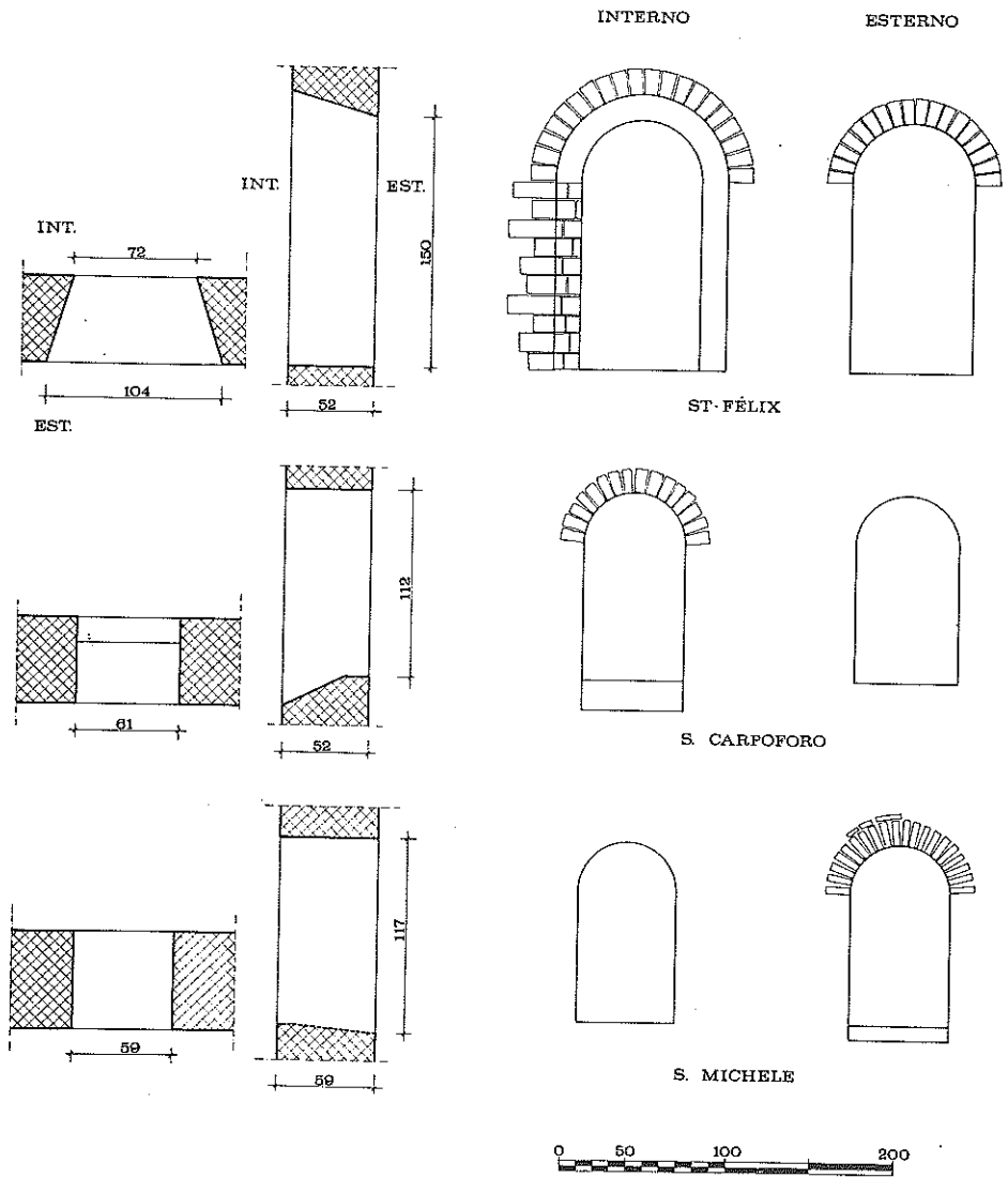
Fig. 56 - Raffronto tra le finestre delle tre chiese.
