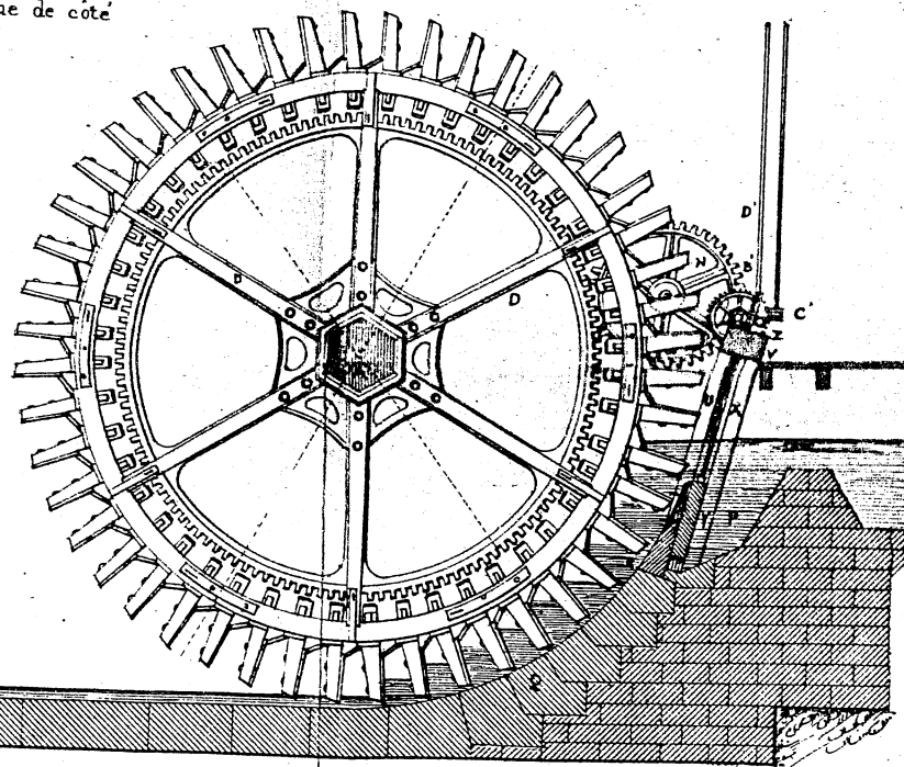
Fig. 3. Vue de côté
