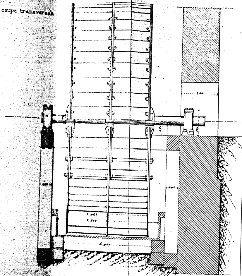
Fig. 4. Elevation & Coupe
