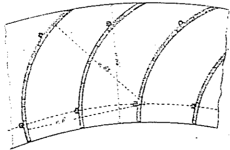
B. Coupe et détails de construction des tubes. Fig. 2.
